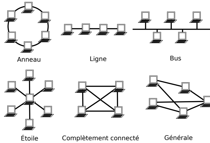
FIGURE 5.7 : Topologies typiques des réseaux numériques.
